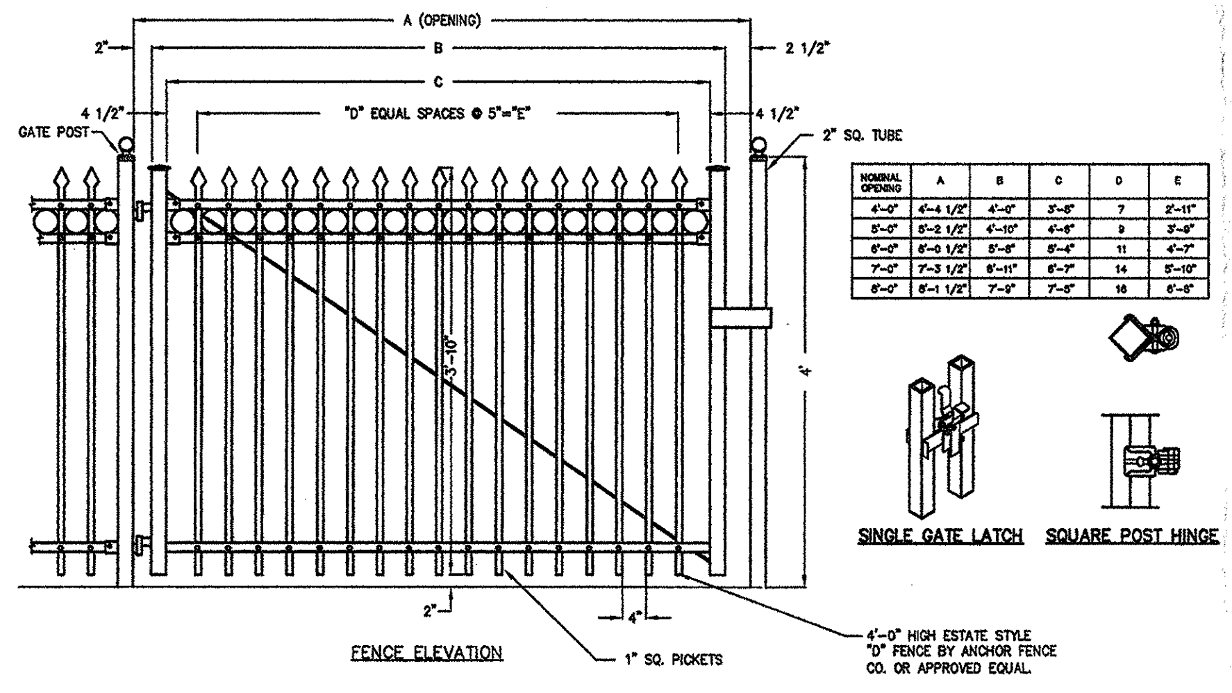
GATE DETAIL N.T.S.
