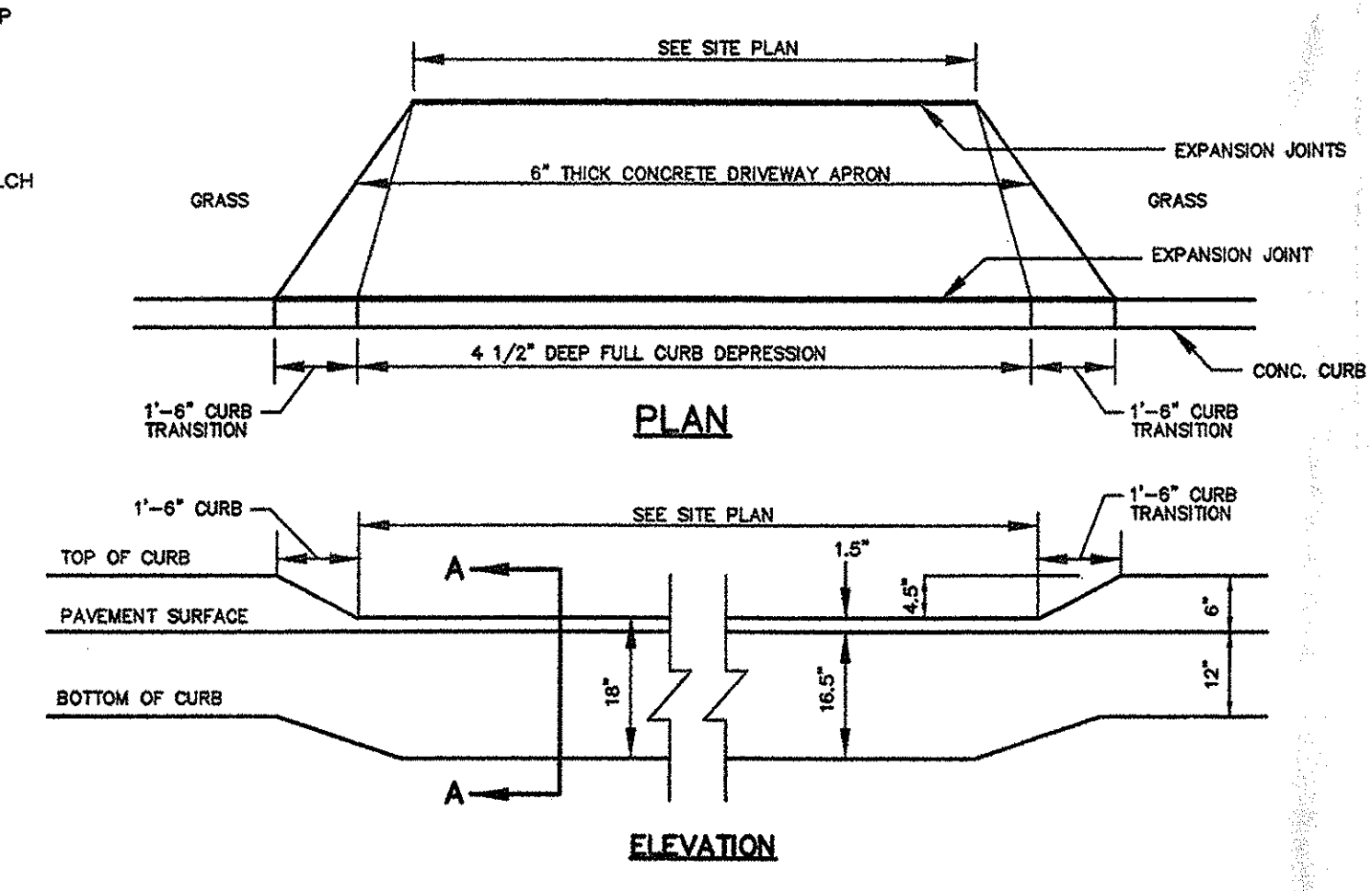
DRIVEWAY APRON & CURB DEPRESSION DETAIL N.T.S.
