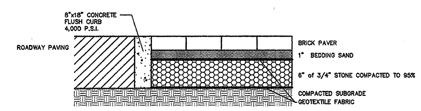
PAVER CROSS SECTION N.T.S.
