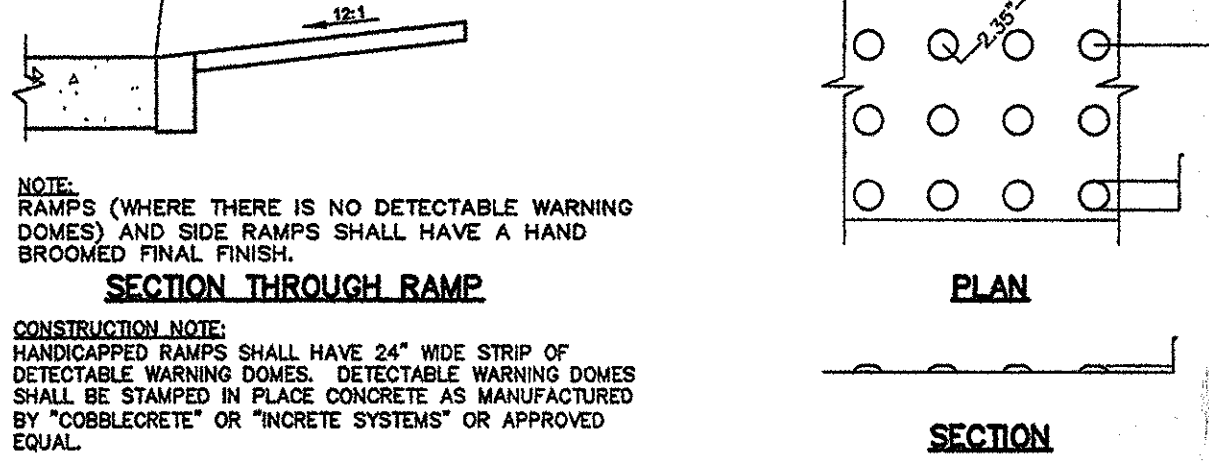
DETECTABLE WARNING DOMES N.T.S.
