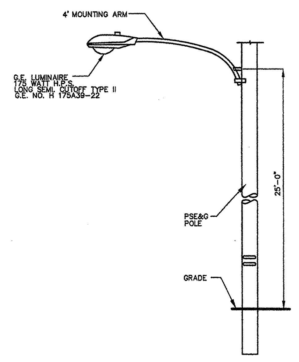
LIGHT DETAIL N.T.S.
