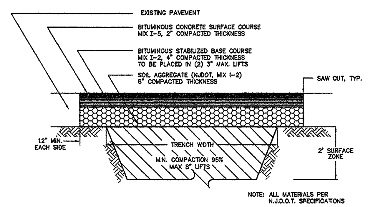
TRENCH & ROADWAY REPAIR DETAIL N.T.S.
